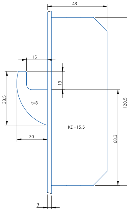
Nebenschloss mit Schwenkriegel
