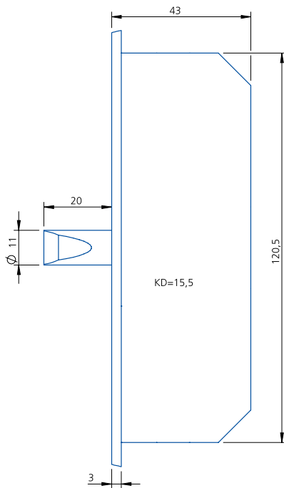
Nebenschloss mit Bolzenriegel
